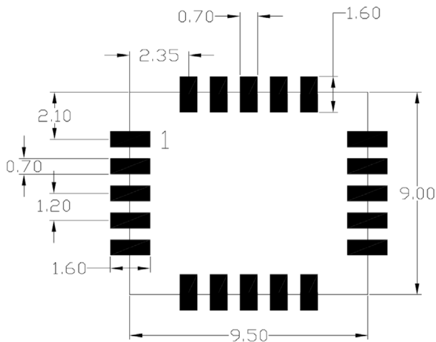
Fig. 2.2 PCB pad
