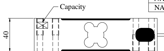
主視(Front View)
